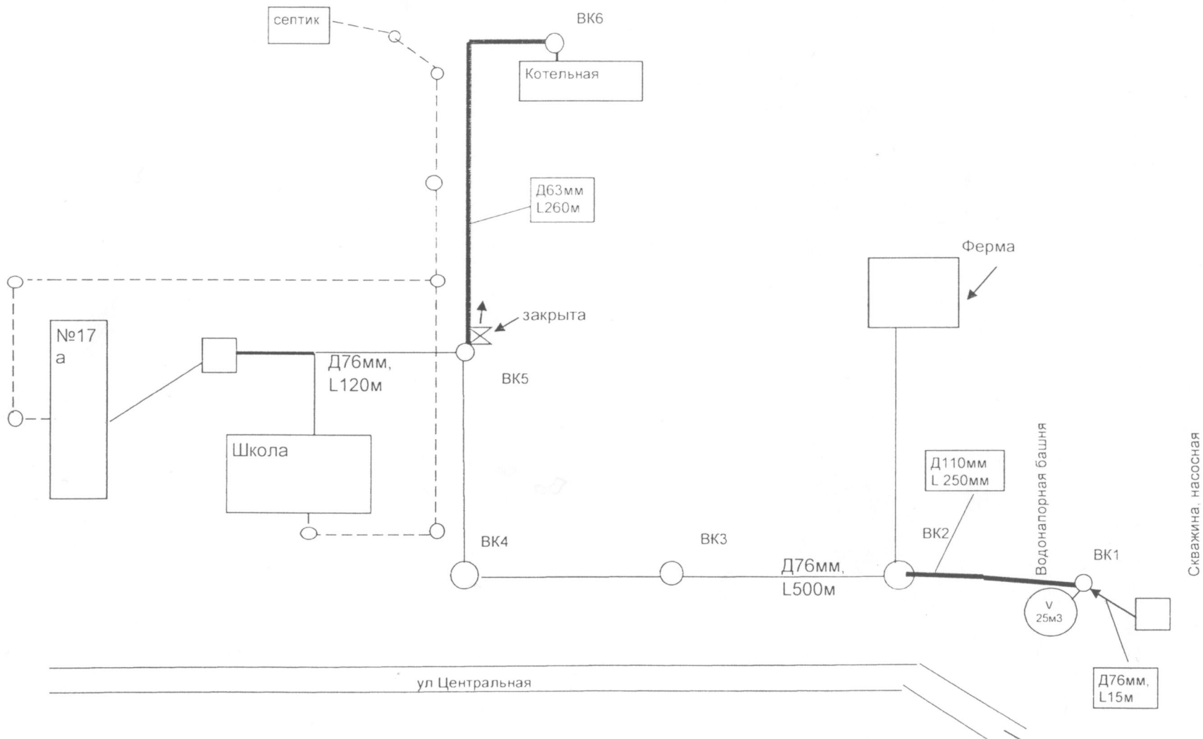
Схема водоснабжения и канализации. Устиновка
