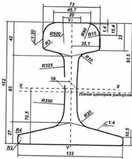
Рис.1 Рельс Р 50
